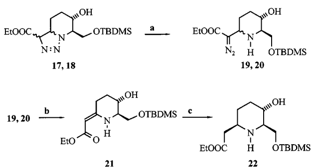
Scheme 6. a) i. \text{Et}_3\text{N} , \text{CH}_2\text{Cl}_2 , 12 h, 96%; b) \text{Rh}_2(\text{OAc})_4 , 12 h, 97%; c) \text{H}_2 , 10% Pd/C, EtOH, 48 h, 71%
