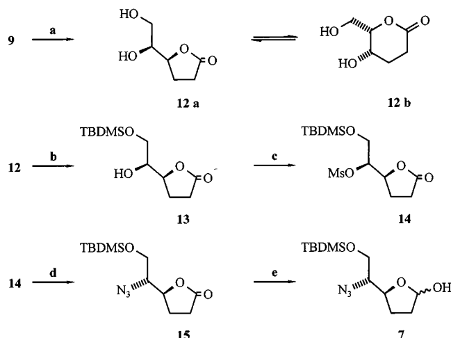
Scheme 3. a) concd. HCl, i PrOH, 48 h, 96%; b) excess TBDMSCl, Et 3 N, DMAP, DMF, 12 min, 99%; c) MsCl, Et 3 N, CH 2 Cl 2 , 20 min, 79%; d) NaN 3 , DMPU, 70^\circ\text{C} , 24 h, 65%; e) DIBALH, THF, -78^\circ\text{C} , 4–6 h, 69%
